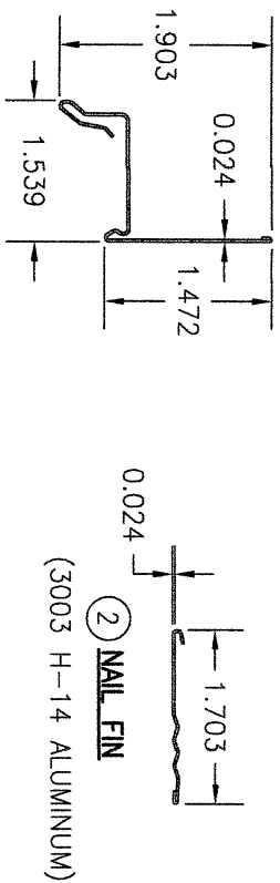
① DRIP CAP NAIL FIN (3003 H-14 ALUMINUM)
